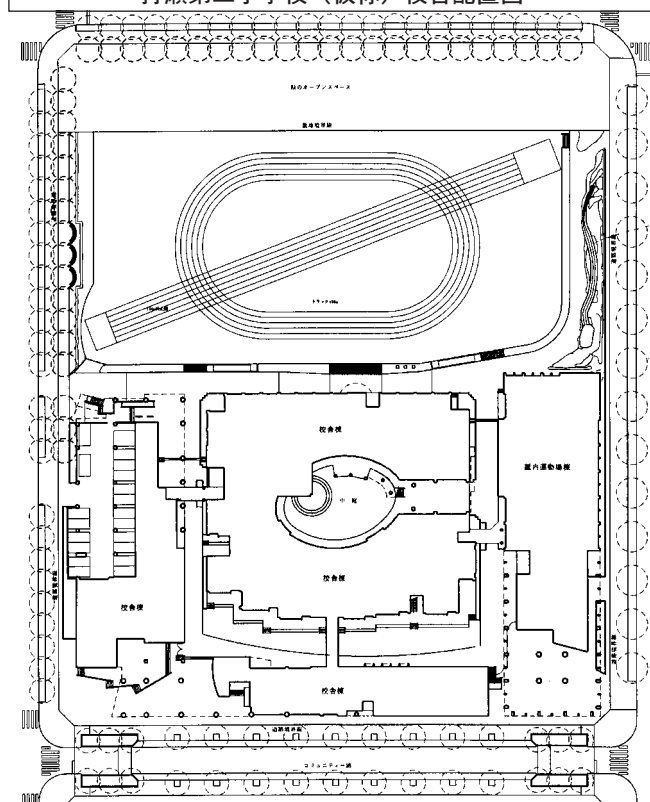
打瀬第二小学校（仮称）校舎配置図
